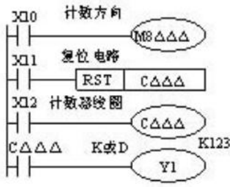
图 7 高速计数器的使用
