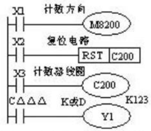
图 5 32 位双向计数器的使用
