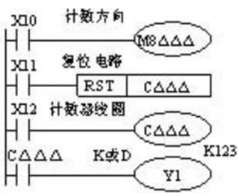
图 6 高速计数器的使用
